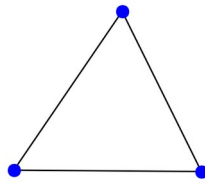
K_3
